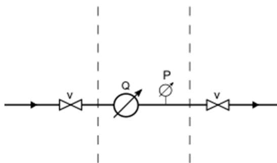
Rys. 10 Schemat montażu urządzeń pomiarowych. (Q - wodomierz/przepływomierz, p - czujnik ciśnienia, v - zasuwka).
