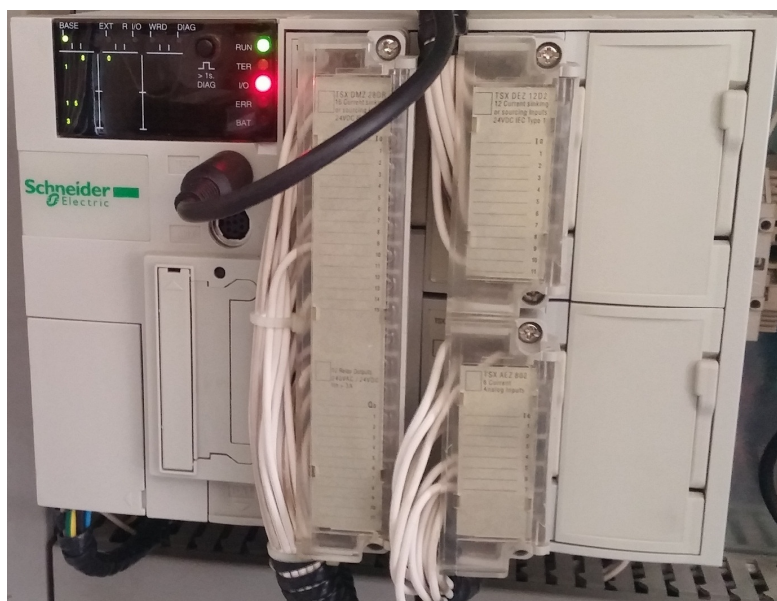
Rys. 6 Sterownik TSX Micro sterujący centralną hydrofornią.
